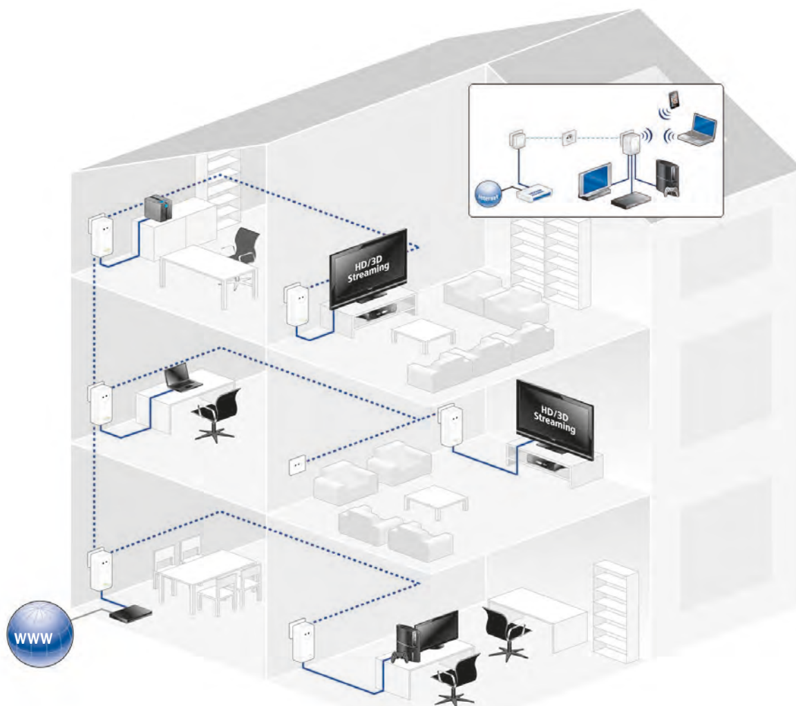
Heimnetzwerk über dLAN® mit bis zu 500 MBit/s für Full HD Übertragung Foto: devolo.de
